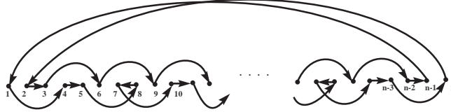
Fig. 24. T_n\langle 1, 3; 1, 2m \rangle ; n = 2m + 2 where 2m \equiv 0 \pmod 3 .
